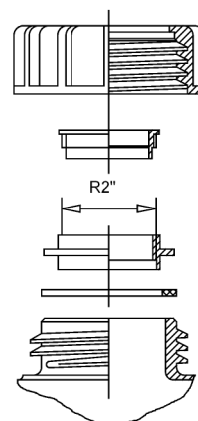
Detalj-Gånganslutning
