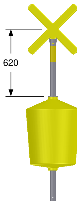
Markeringsboj 100 L
